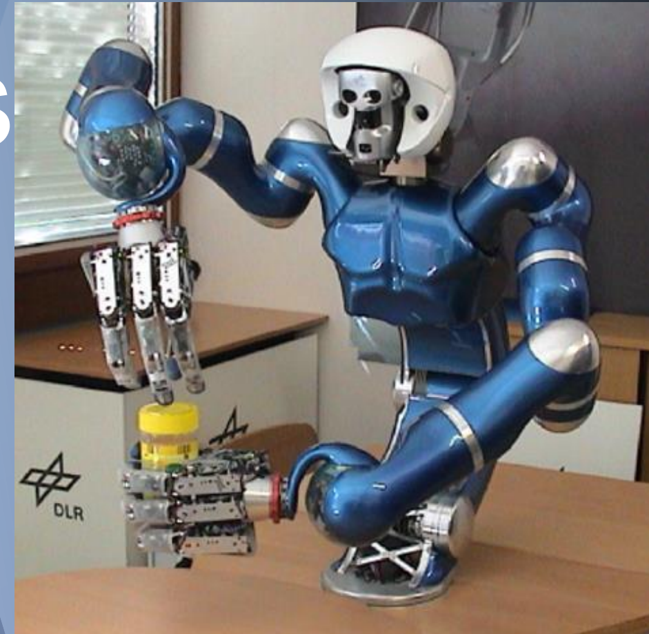
The DLR Humanoid Manipulator Justin www.dlr.de/rm
